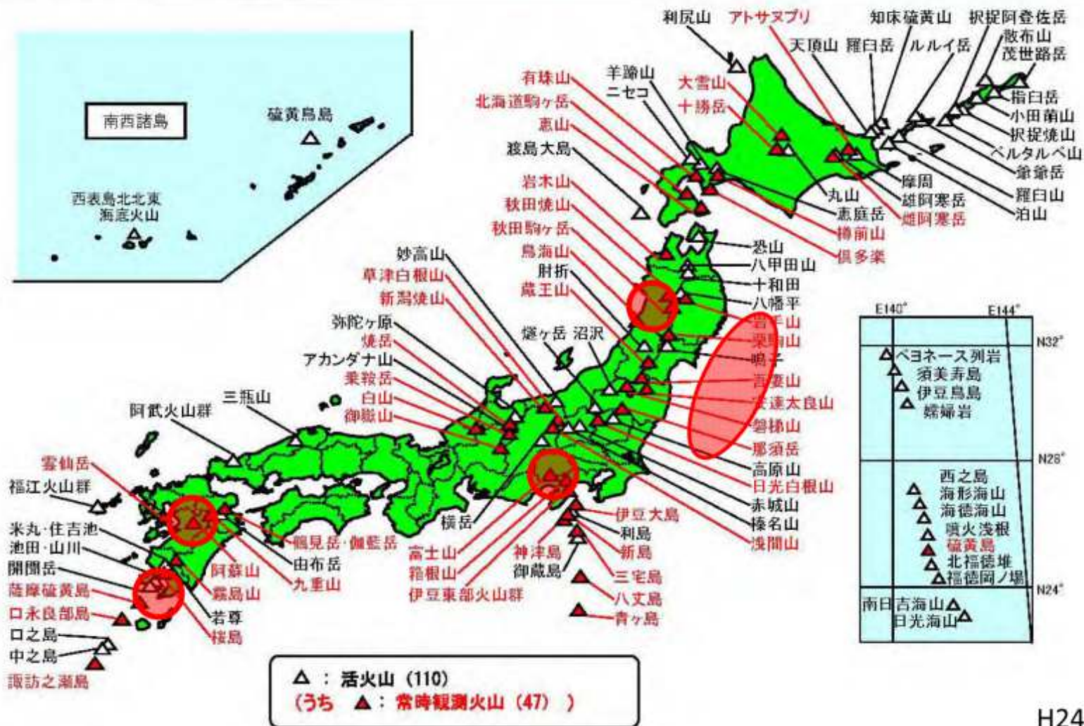
図表 1-2-11 日本の活火山分布
